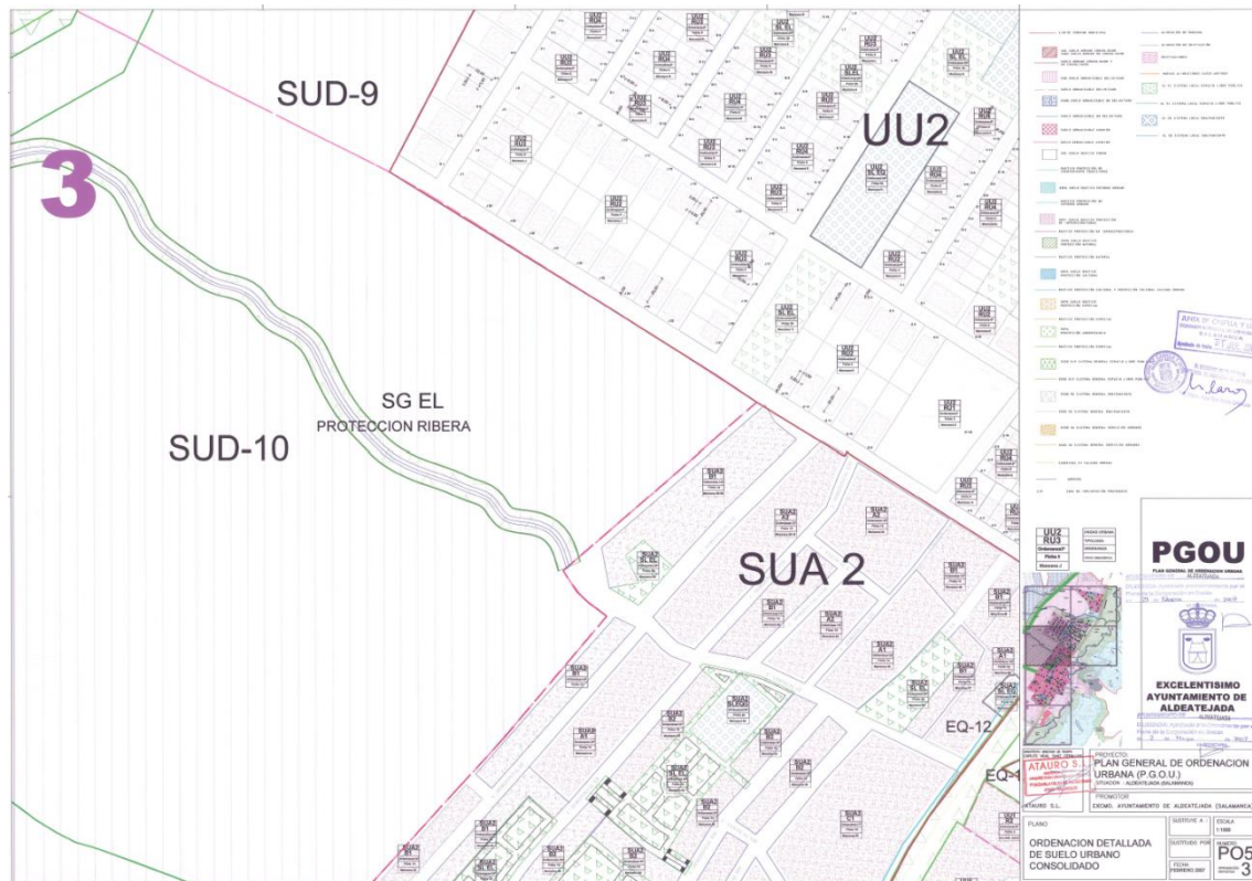
Figura 6: Plano PO5.3. Ordenación Detallada de Suelo Urbano Consolidado del PGOU (Fuente: http://www.jcyl.es/ )
