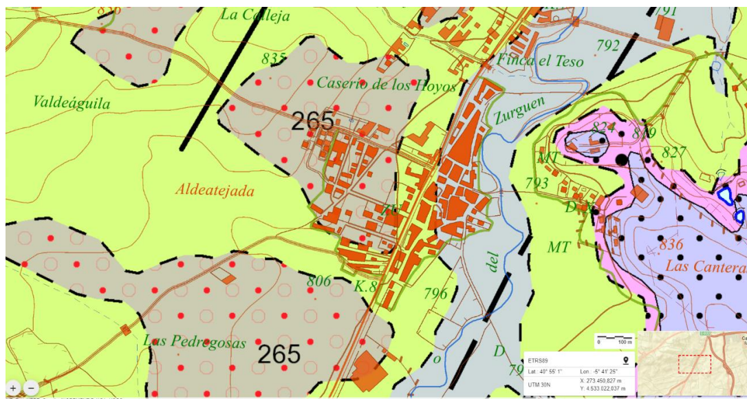
Figura 3: Mapa geológico del Sector y su entorno (Fuente: http://info.igme.es/ )
